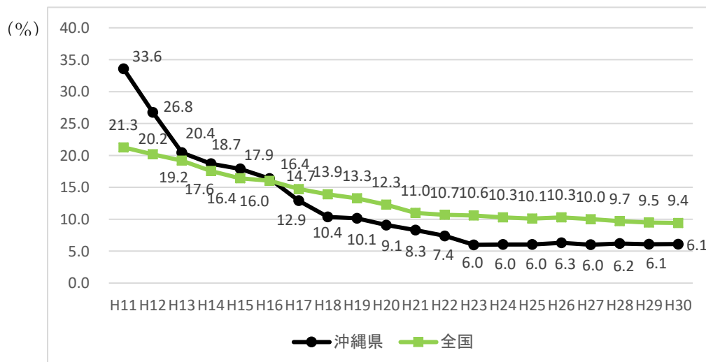
図 2 - 7 最終処分率の推移
