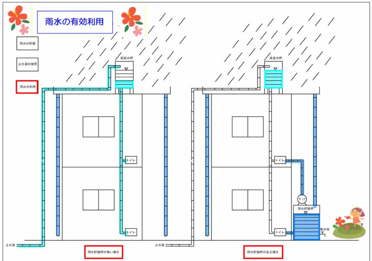
図IV-3-1 製作する雨水利用の模型パネル (イメージ)
