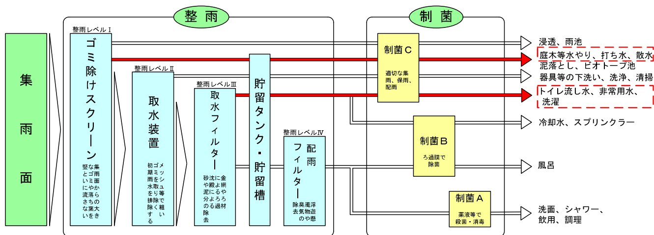
整雨・制菌フロー
