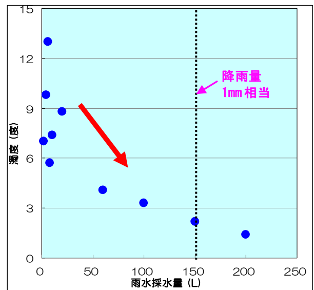
初期雨水の雨量と濁度の変化
