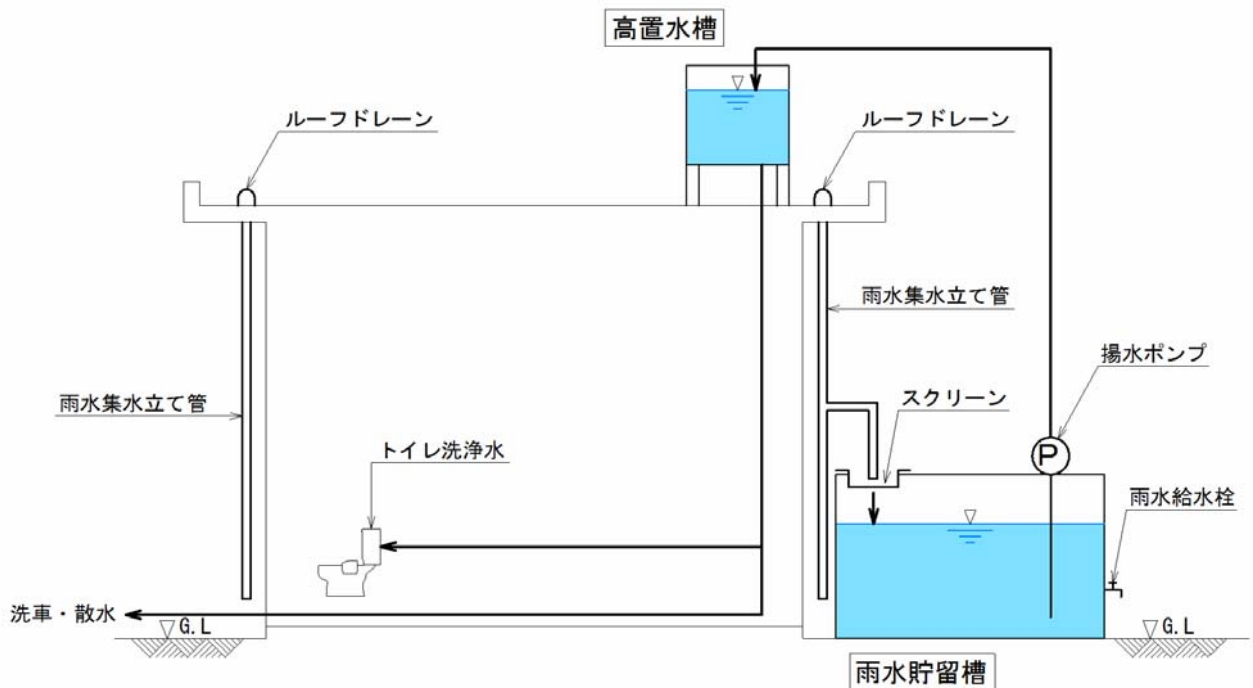
雨水利用システムの例（地上設置型）
