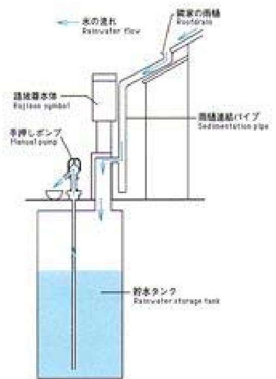
路地尊の構造
