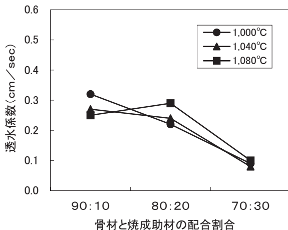
図6 成形圧3.9MPaとした時の透水係数の変化
